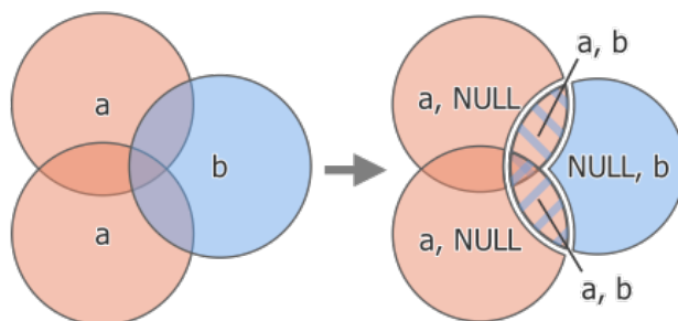
Fig. 24.129: Unionsoperation mellan ett inmatningslager med två funktioner "a" och ett överlagringslager med en funktion "b" (vänster) - resulterande lager med fem funktioner med attribut från båda lagren (höger)
