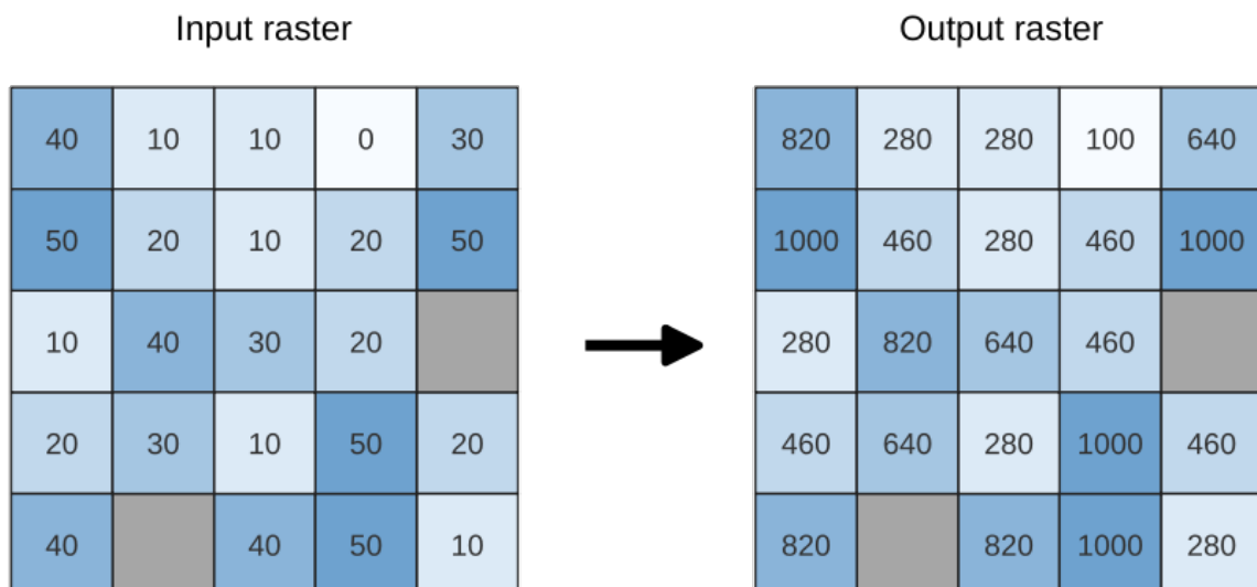
Fig. 24.26: Omskalning av värden för ett rasterlager från [0 - 50] till [100 - 1000]
