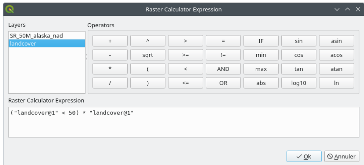
Fig. 13.24: Kalkylator för rasteruttryck
