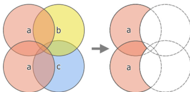
Fig. 24.120: Skillnadsoperation mellan ett inmatningslager med två funktioner "a" och överlagringslager med en funktion "b" och "c" (vänster) - resulterar i ett nytt lager med de modifierade funktionerna "a" (höger)
