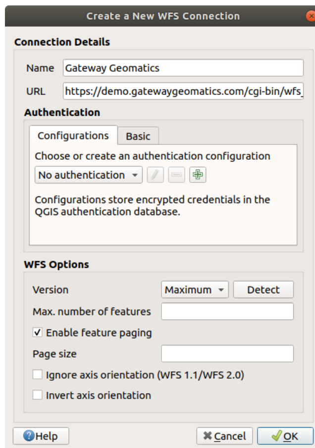
Fig. 19.6: Skapa en anslutning till en WFS-server
