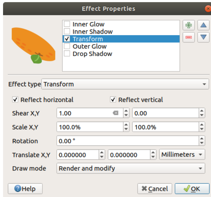
Fig. 12.24: Rita effekter: Dialogrutan Transformera
