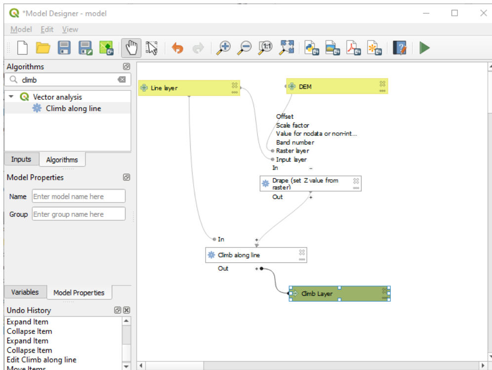
Fig. 23.24: En komplett modell
