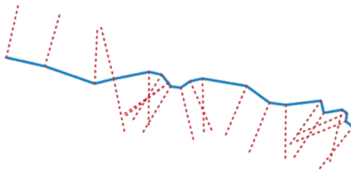
Fig. 24.114: Streckade röda linjer representerar transekten för det ingående linjelagret
