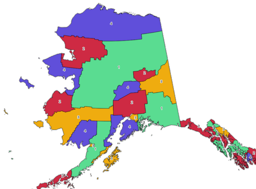
Fig. 24.1: Exempel på topologiska färger
