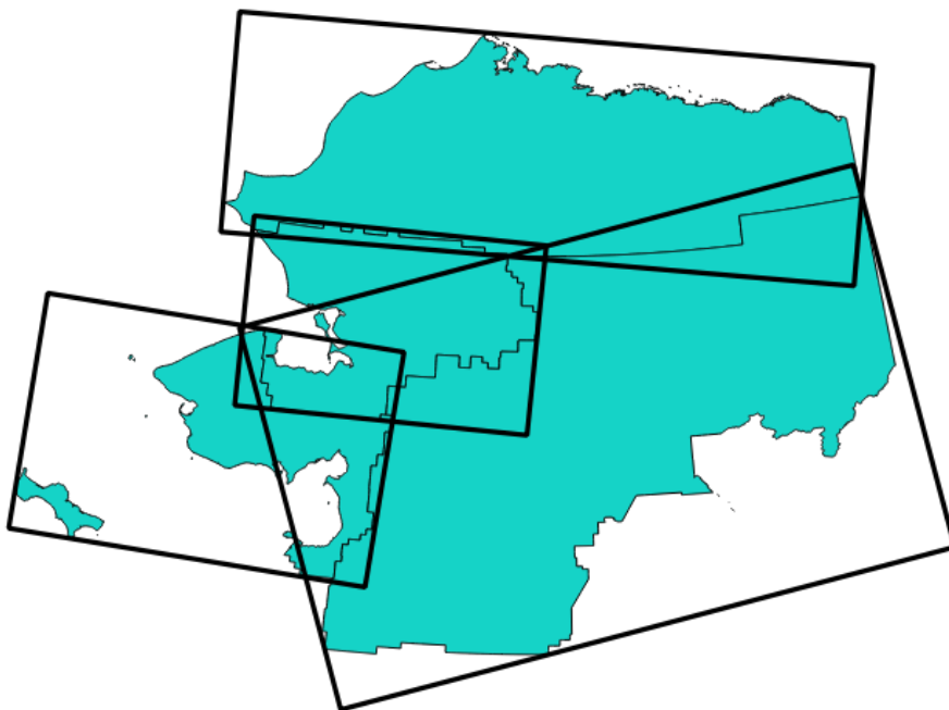
Fig. 24.97: Orienterad minsta avgränsande box
