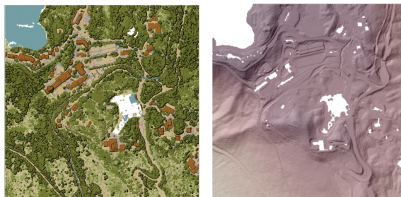
Fig. 24.11: Terrängraster som genereras genom triangulering av punktmoln
