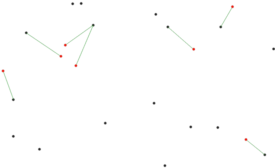
Fig. 24.40: Visa närmaste hubb för de röda inmatningsfunktionerna
