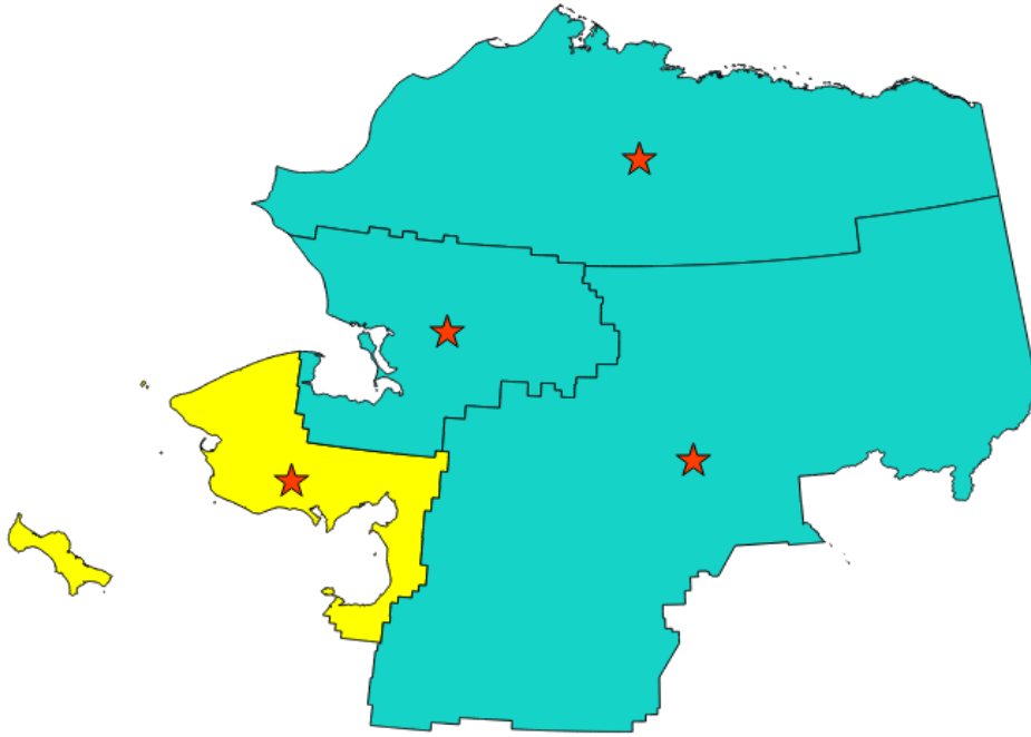
Fig. 9.9: De röda stjärnorna representerar centroiderna för funktionerna i inmatningslagret.
