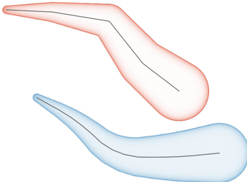
Fig. 9.34: Avsmalnande buffert på linjefunktioner
