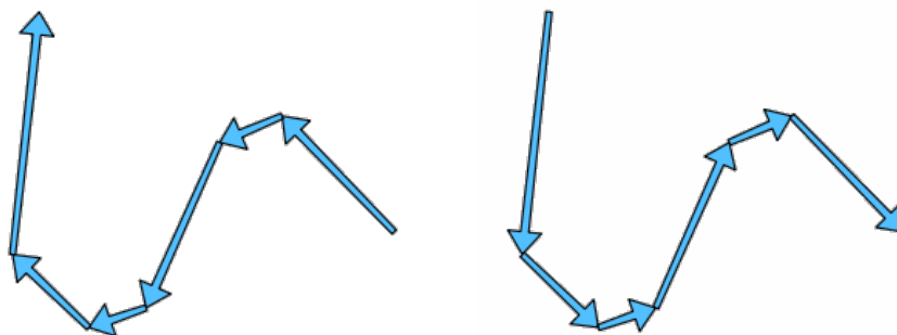
Fig. 9.26: Vändning av linjens riktning
