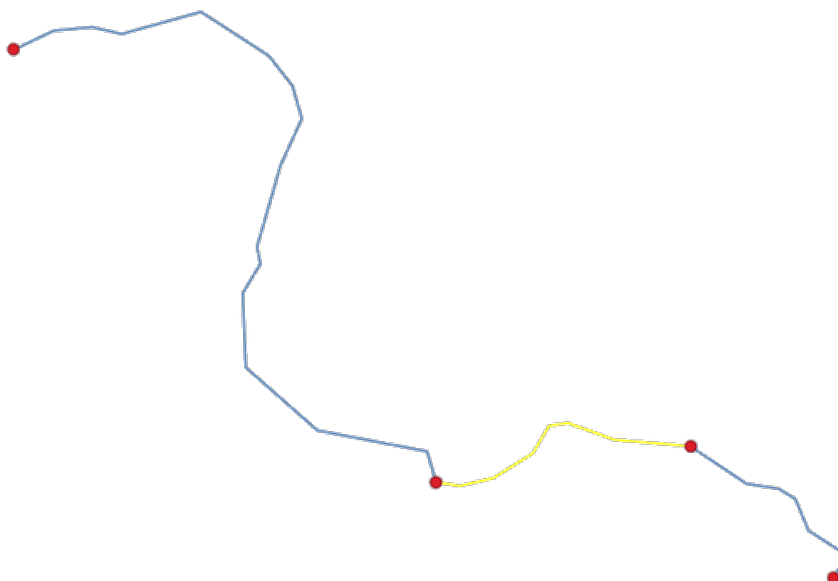
Fig. 24.60: Gränsskikt (röda punkter) för linjer. I gult en vald funktion.
