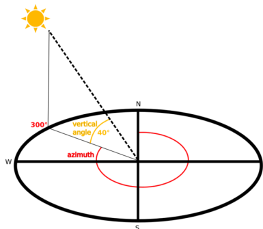
Fig. 24.31: Azimut och vertikal vinkel
