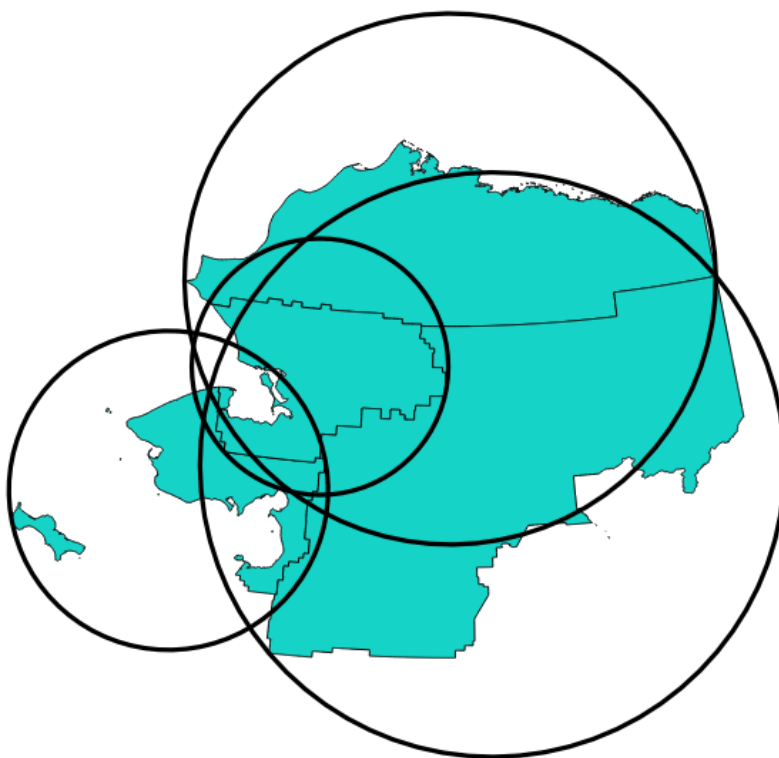
Fig. 9.21: Minimal omslutande cirkel för varje funktion
