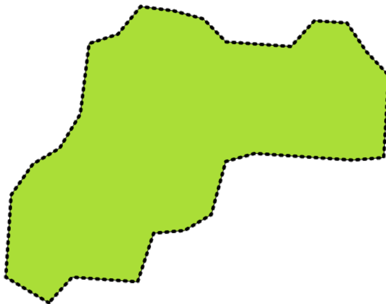
Fig. 24.59: Gränser (svart streckad linje) för källans polygonlager
