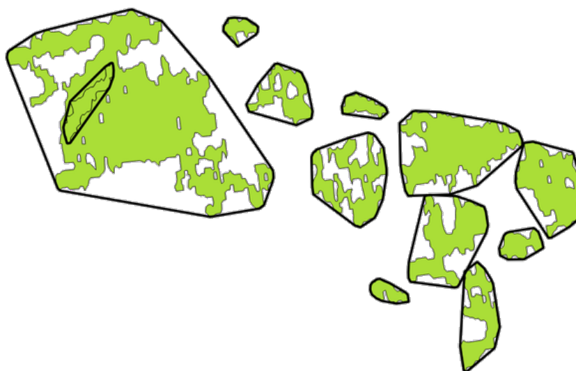
Fig. 9.11: Svarta linjer identifierar det konvexa skrovet för varje funktion
