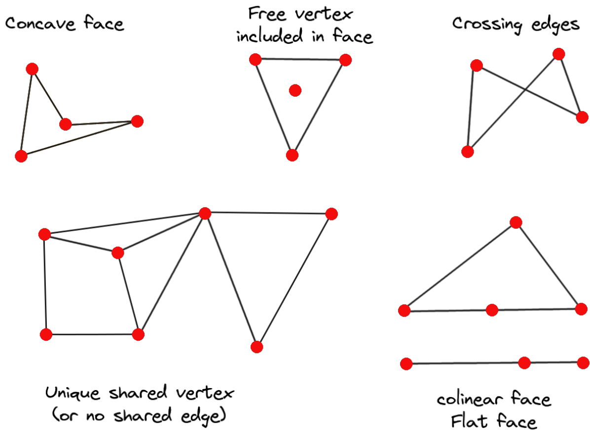
Fig. 14.16: Exempel på ogiltiga maskor
