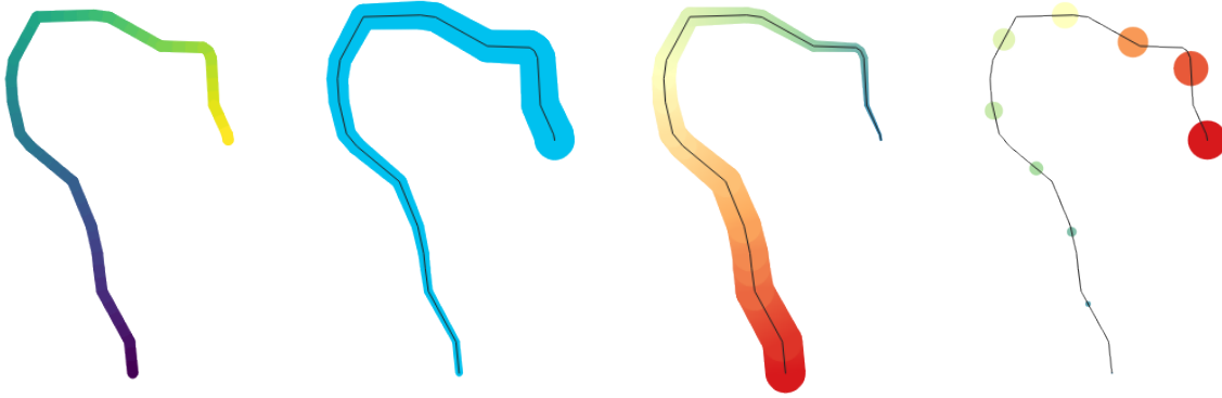
Fig. 10.13: Exempel på interpolerade linjer
