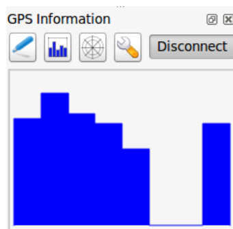
Fig. 20.4: Signalstyrka för GPS-spårning
