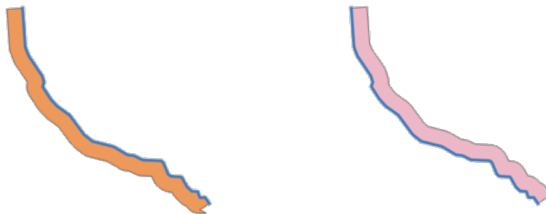
Fig. 9.29: Vänster- och högersidig buffert på samma vektorlinjelager
