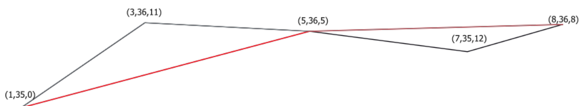
Fig. 24.86: Den röda linjen representerar den svarta linjen med endast toppar vars Z-värde är \leq 10 .
