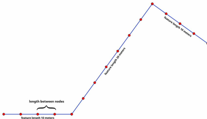
Fig. 24.77: Förtäta geometrin vid ett givet intervall
