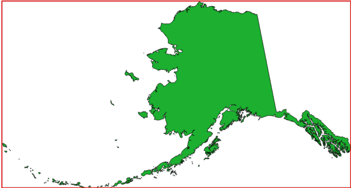
Fig. 24.7: I rött avgränsningsrutan för källlagret
