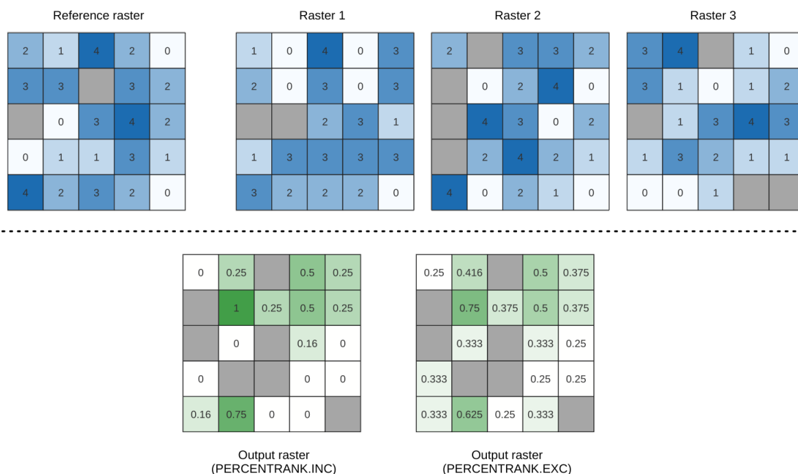
Fig. 24.18: Procentuell ranking Värde = 1. NoData celler (grå) ignoreras.
