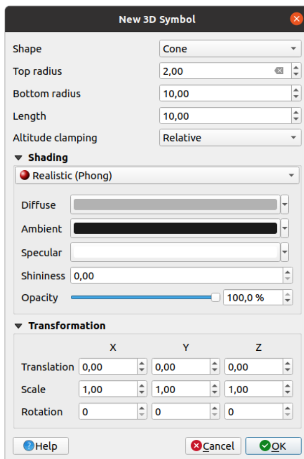
Fig. 10.36: Egenskaper för en 3D-punktsymbol
