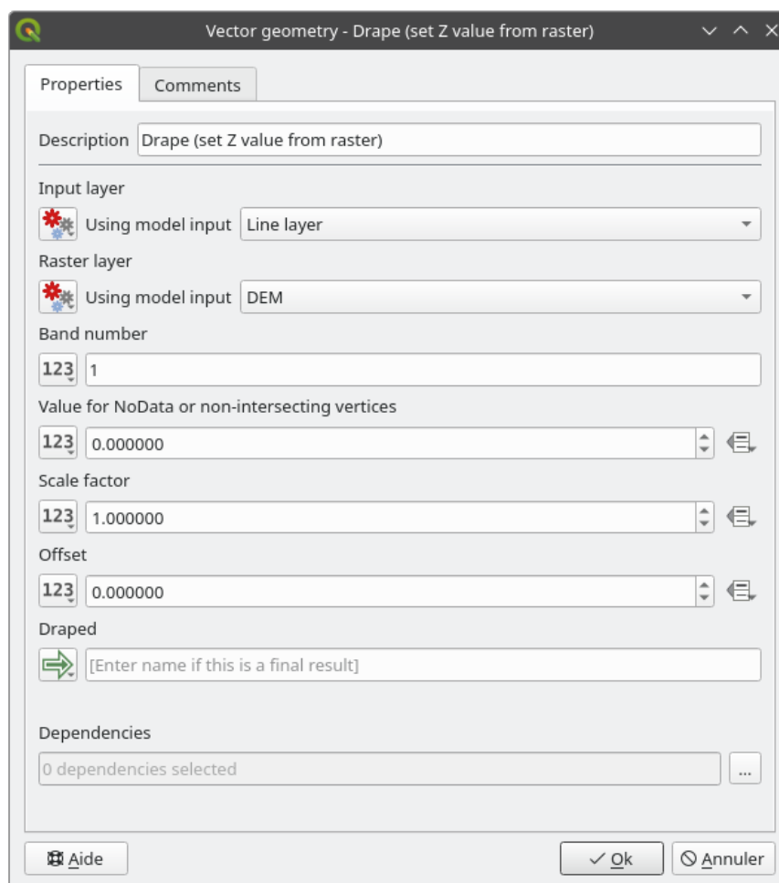
Fig. 23.23: Algoritm Parametrar för inmatning och utmatning
