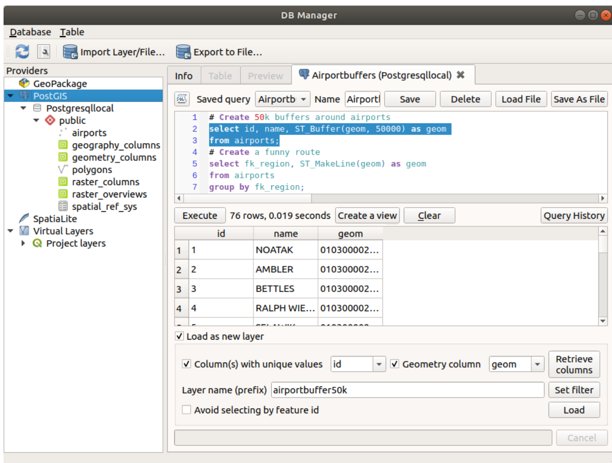
Fig. 25.5: Exekvera SQL-frågor i SQL-fönstret i DB Manager
