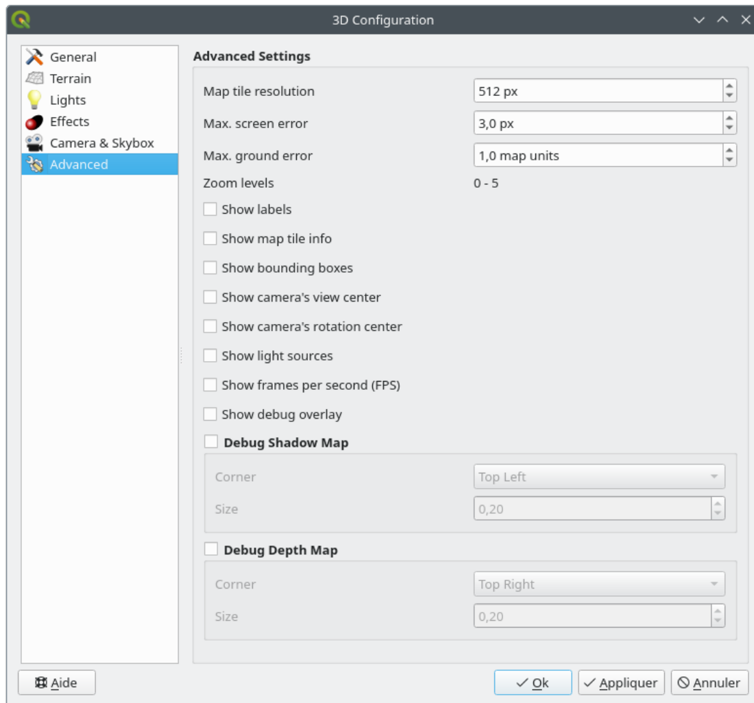
Fig. 7.30: Dialogrutan Avancerad konfiguration för 3D-karta
