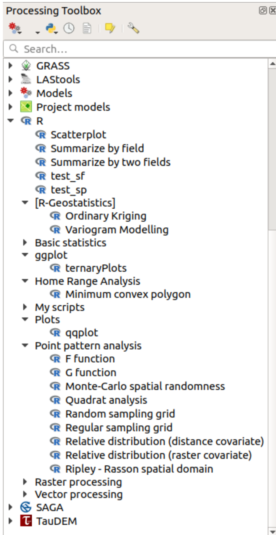
Fig. 23.35: Verktygslådan Processing Toolbox med några R-skript som visas
