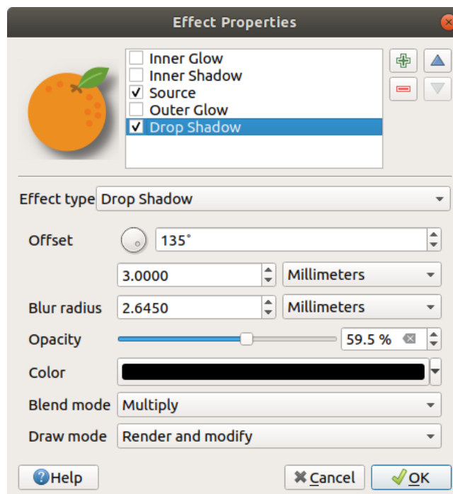
Fig. 12.20: Rita effekter: Dialogrutan Drop Shadow
