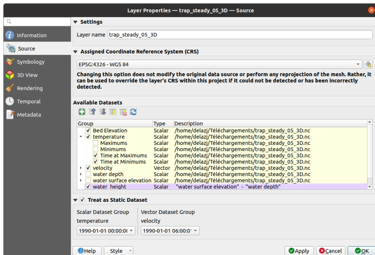
Fig. 14.5: Egenskaper för Mesh Layer Source
