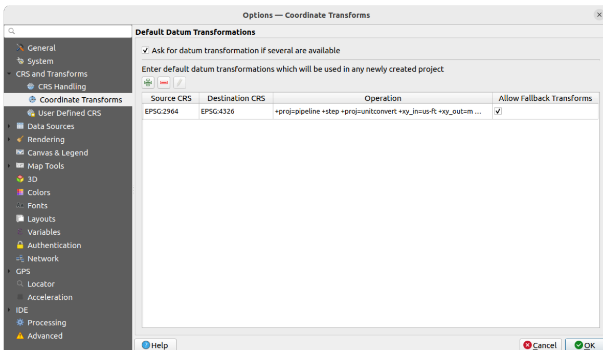
Fig. 5.4: Inställningar för transformationer
