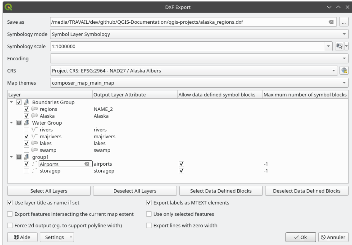
Fig. 11.32: Exportera ett projekt till DXF-dialogrutan
