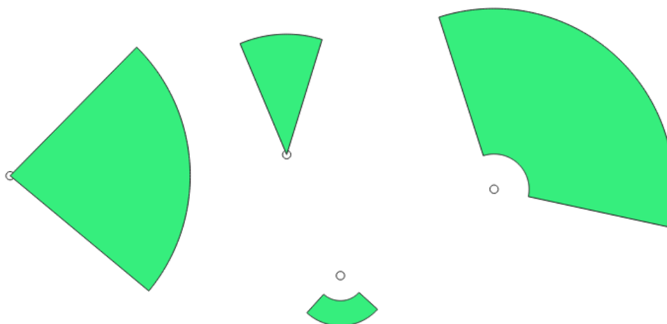
Fig. 9.40: Funktioner för buffring av kilar
