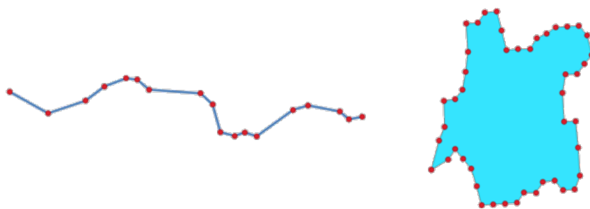
Fig. 24.84: Extraherade hörnpunkter för linje- och polygonlager
