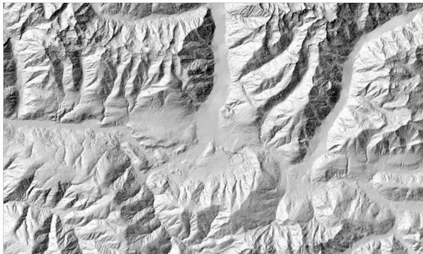
Fig. 24.32: Terrängskuggningslager med azimuth 300 och vertikal vinkel 45
