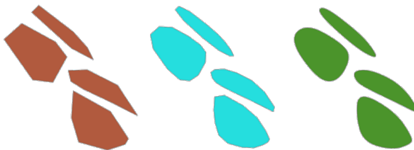
Fig. 24.109: Ökat antal iterationer ger jämnare geometrier
