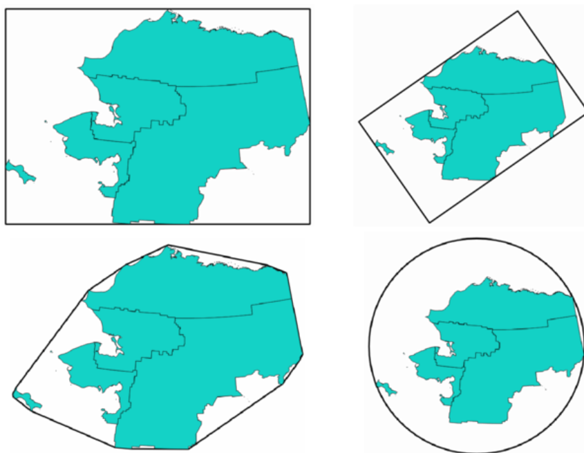
Fig. 24.90: Medurs från övre vänstra hörnet: kuvert, orienterad rektangel, cirkel, konvex kropp
