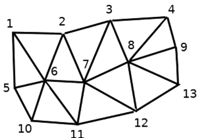
Fig. 14.2: Triangulärt rutnät med numrerade hörn
