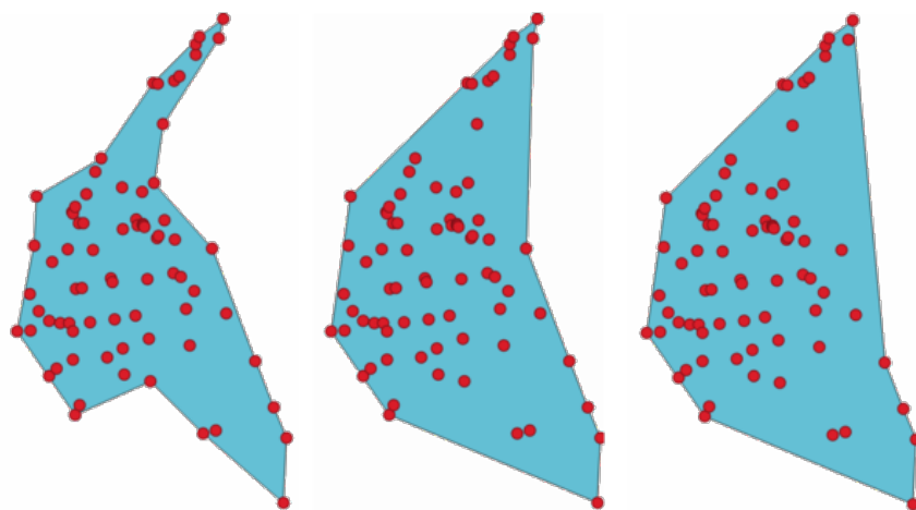
Fig. 24.70: Konkava skrov med olika tröskelvärden (0,3, 0,6, 0,9)
