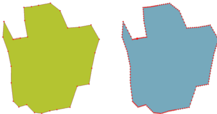
Fig. 9.12: Röda punkter visar topparna före och efter förtätningen
