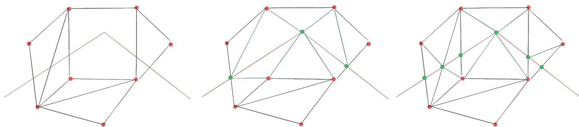
Fig. 14.17: Force Mesh med linjegeometri - Resultat utan (mitten) och med (höger) ny vertex på kanternas skärningspunkt
