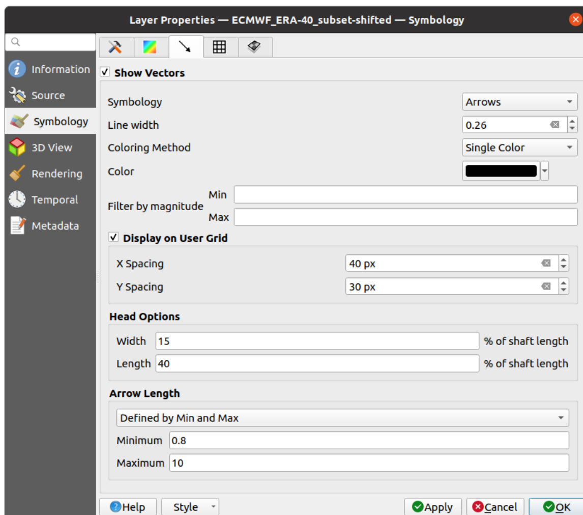
Fig. 14.8: Styling av vektorer i ett mesh-lager med pilar
