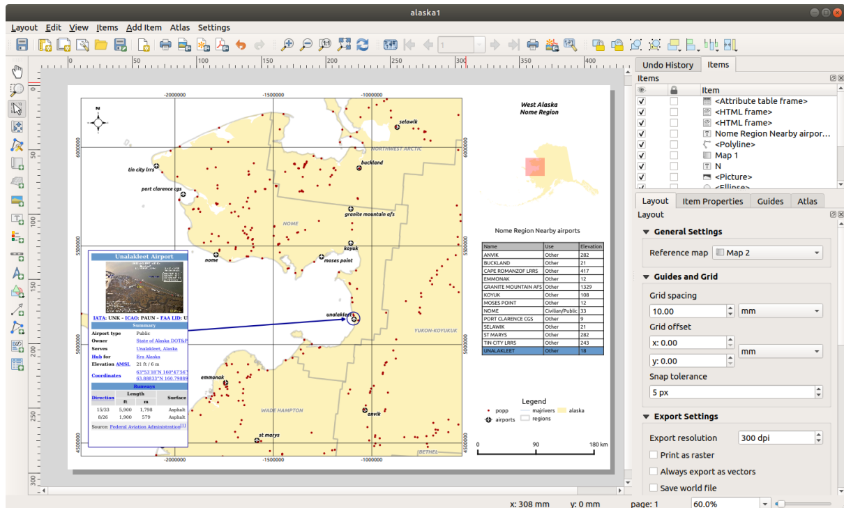
Fig. 18.63: Utskriftslayout med kartvy, teckenförklaring, bild, skalstreck, koordinater, text och HTML-ram tillagd
