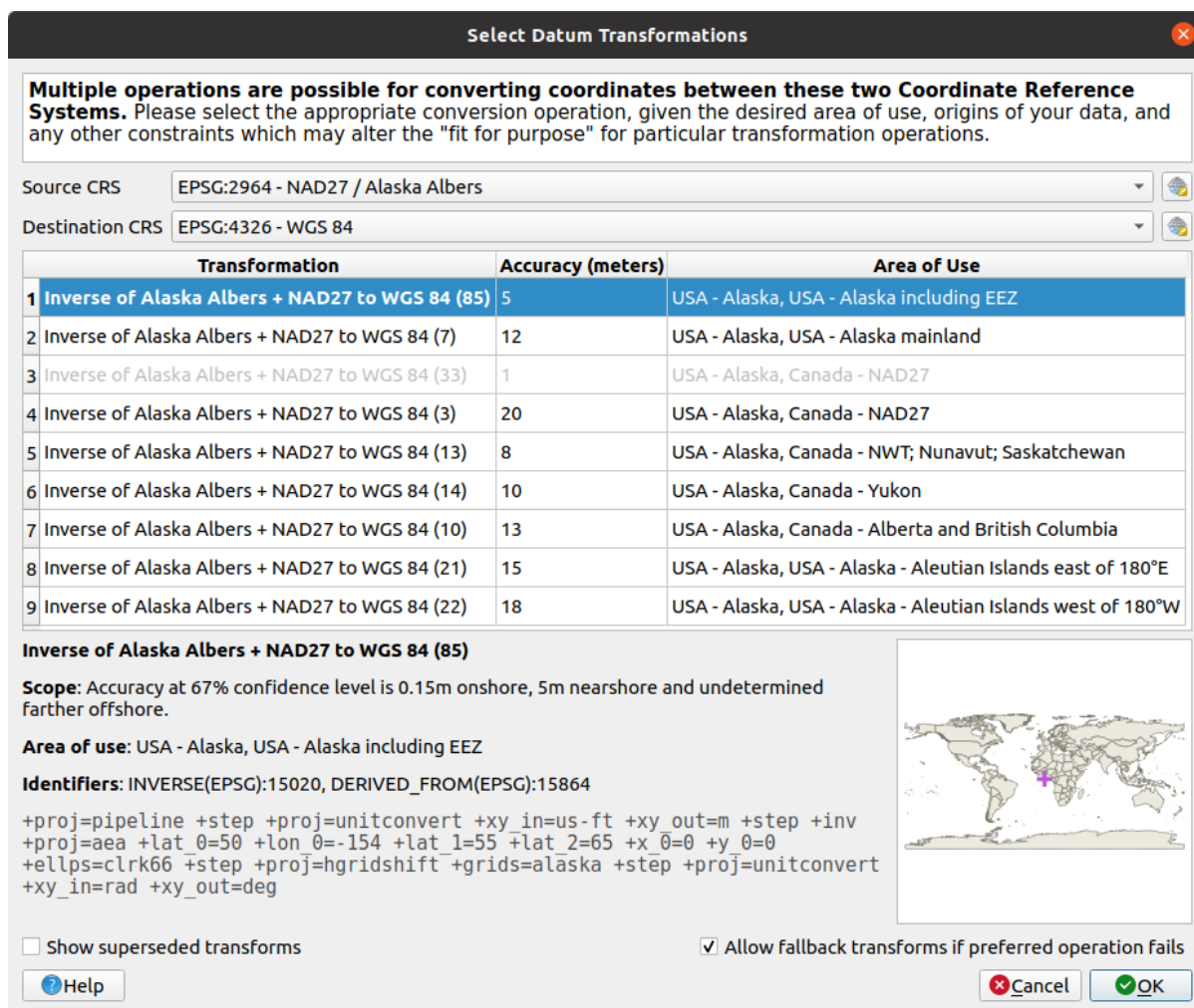
Fig. 6.6: Val av en föredragen standard datumtransformation
