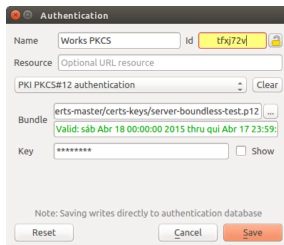
Fig. 21.34: Ändra ett lagets konfigurations-ID för autentisering (olåst gult textfält)
