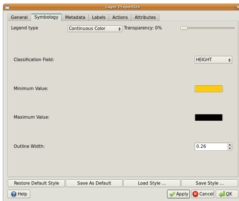
Fig. 4.11: Konfigurera kontinuerlig färgsymbologi. Attributet konturhöjd används för att bestämma färgvärden. Färger definieras för minimi- och maximivärdena. GIS-applikationen skapar sedan en färggradient för att rita objekten baserat på deras höjder.
